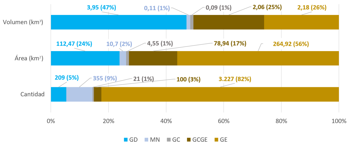
FIG. 10. Comparación entre la cantidad de geoformas mapeadas, su área (km²) y su volumen estimado de agua equivalente (km³).
