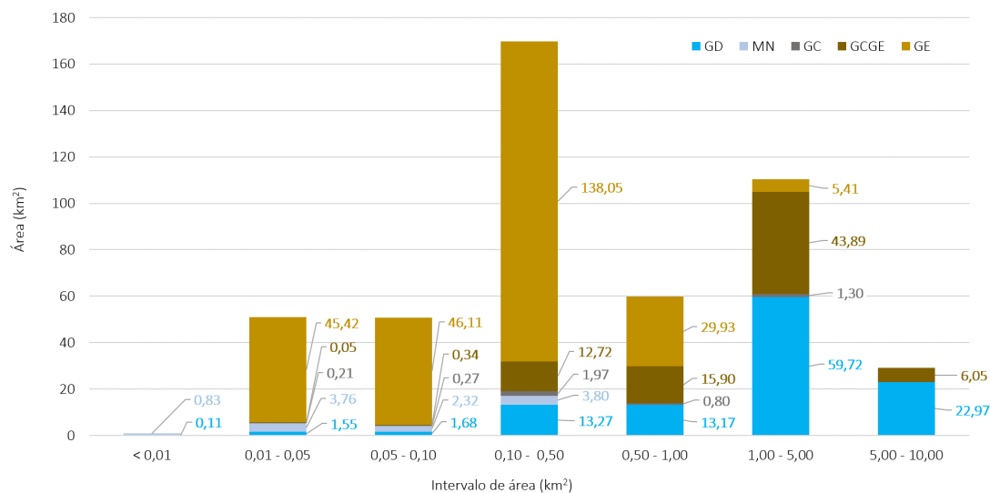
FIG. 3. Área acumulada de geoformas inventariadas discriminadas por intervalo de área y tipo de geoforma. Abreviaciones según figura 2.
