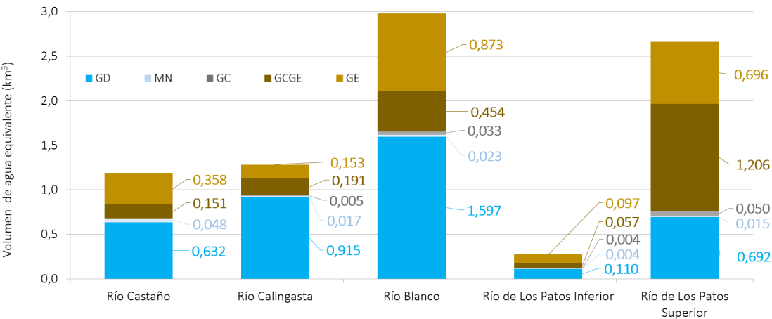
FIG. 9. Volumen de agua equivalente (km³), desglosado según tipo de geoforma y subcuenca.
