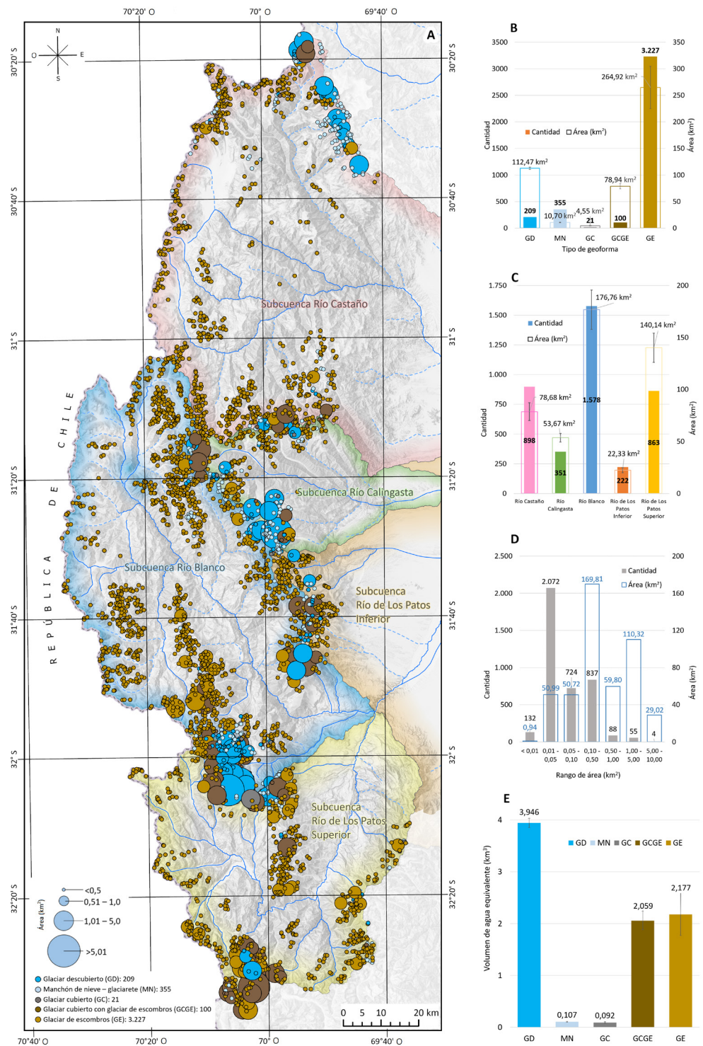
FIG. 2. A. Ubicación de las geoformas inventariadas, agrupadas por tipología y rango de área. B. Cantidad y área de geoformas inventariadas, individualizadas por geoforma. C. Cantidad y área de geoformas inventariadas, individualizadas por subcuenca. D. Cantidad y área de geoformas inventariadas, individualizadas según superficie. E. Volumen estimado de agua equivalente, individualizado por geoforma.
