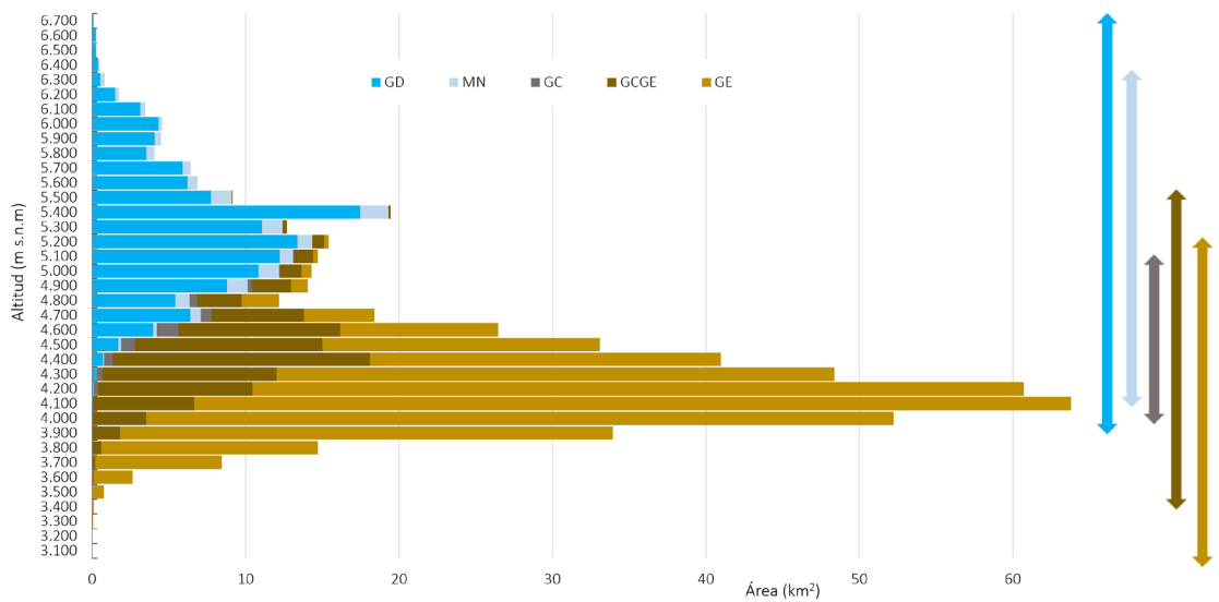
FIG. 4. Hipsometría de geoformas inventariadas, individualizadas según tipo.
