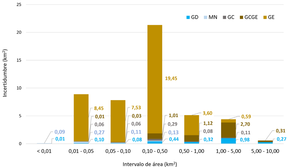
FIG. 8. Distribución de incertidumbre de área según tipo y tamaño de las geoformas.
