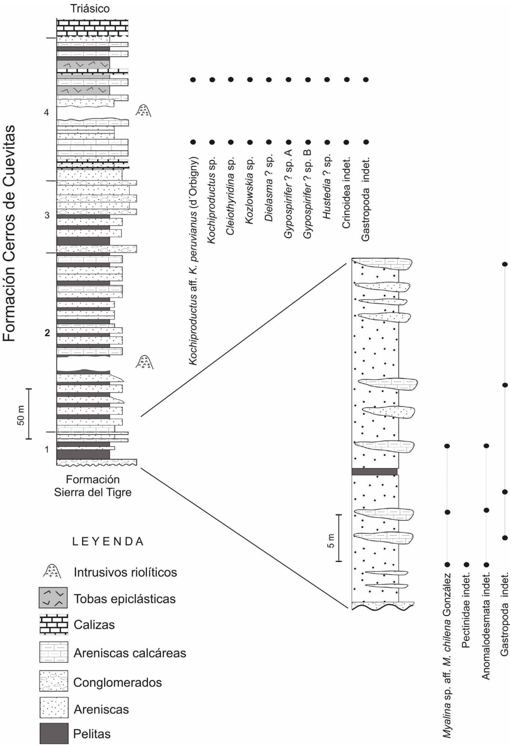
FIG. 3. Sección estratigráfica de la Formación Cerros de Cuevitas, en la localidad homónima, área del salar de Navidad (23°31'34,02"S; 69°57'28,95"W) con los niveles fosilíferos y la distribución vertical de la fauna identificada.
